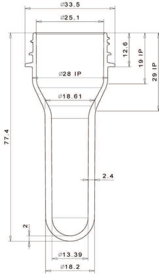
A-A View/Görünüm
